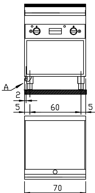
Mod.70/70 FTRG Mod.70/70 FTRG-CR Mod.70/70 FTRRG Mod.70/70 FTRRG-CR
