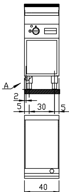
Mod.70/40 FTRG Mod.70/40 FTRG-CR
