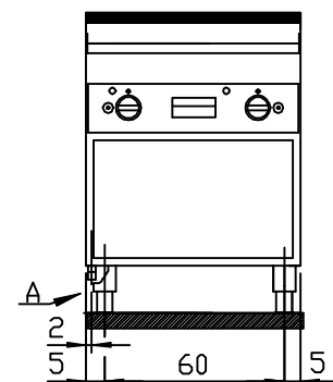
Mod.70/70 FTRG Mod.70/70 FTRG-CR Mod.70/70 FTRRG Mod.70/70 FTRRG-CR
