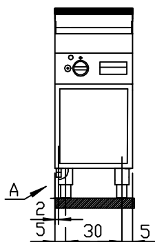
Mod.70/40 FTRG Mod.70/40 FTRG-CR
